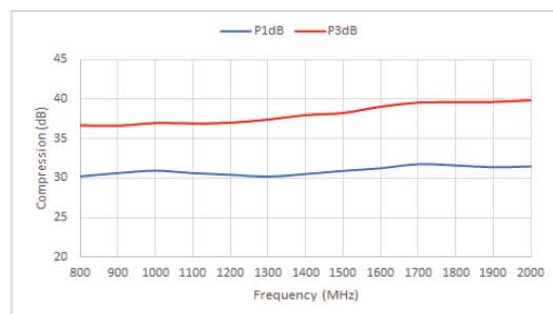
P1dB & P3dB
