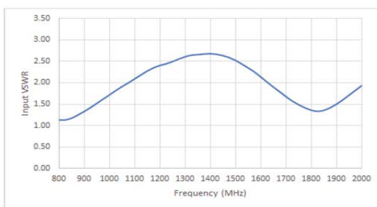
Input VSWR
