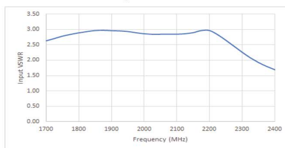
Input VSWR
