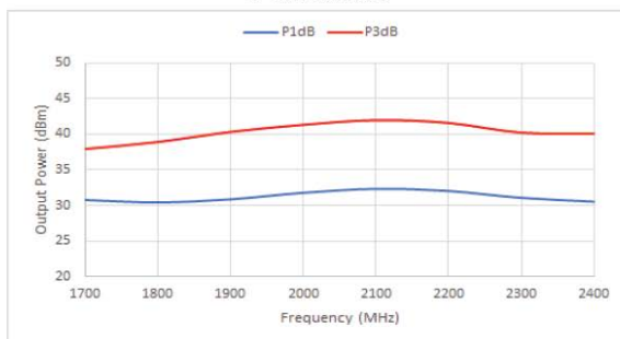
P1dB & P3dB
